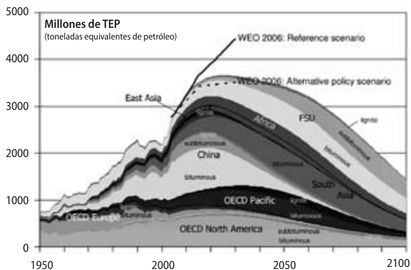
Figura 3. Evolución pasada y posible extracción futura mundial del carbón
