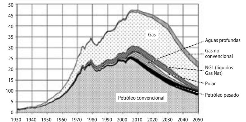
Figura 1. Perfil de la extracción mundial pasada y futura de petróleo y gas natural
